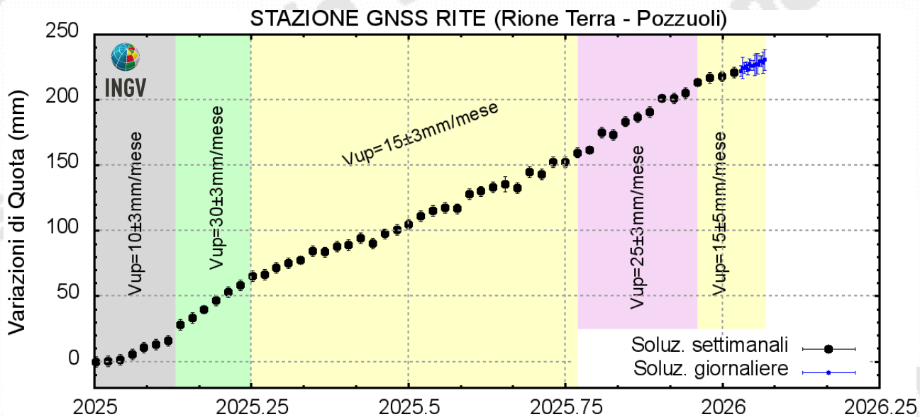
Figura 4.2 – Serie temporale delle variazioni in quota della stazione GNSS di RITE dal 01/01/2025 al 25/01/2026. Elaborazione dati in modalità differenziale singola baseline con software GNSS Spider.
