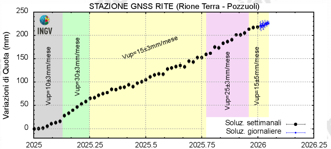
Figura 4.2 – Serie temporale delle variazioni in quota della stazione GNSS di RITE dal 01/01/2025 al 18/01/2026. Elaborazione dati in modalità differenziale singola baseline con software GNSS Spider.
