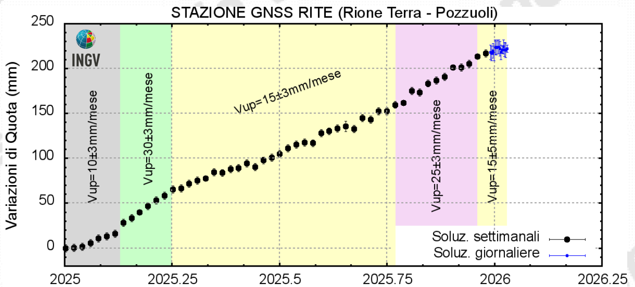
Figura 4.2 – Serie temporale delle variazioni in quota della stazione GNSS di RITE dal 01/01/2025 al 11/01/2026. Elaborazione dati in modalità differenziale singola baseline con software GNSS Spider.
