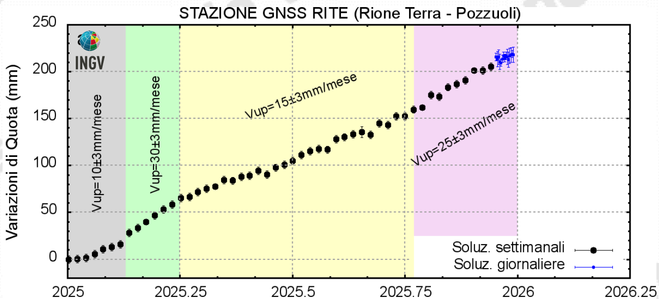
Figura 4.2 – Serie temporale delle variazioni in quota della stazione GNSS di RITE dal 01/01/2025 al 28/12/2025. Elaborazione dati in modalità differenziale singola baseline con software GNSS Spider.
