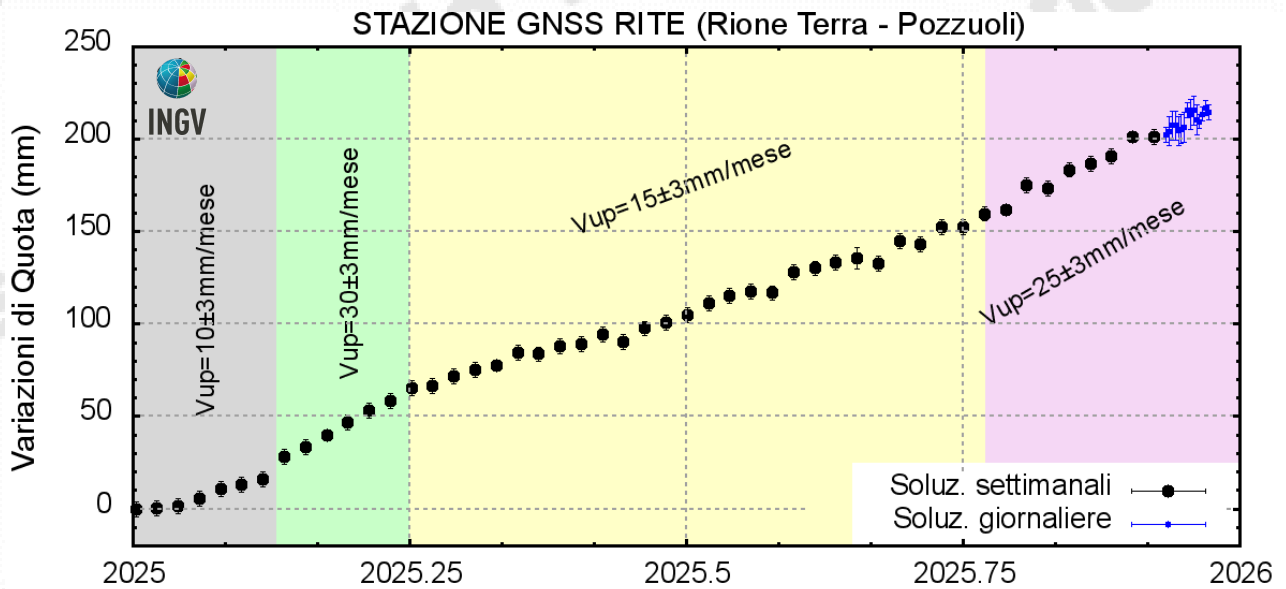
Figura 4.2 – Serie temporale delle variazioni in quota della stazione GNSS di RITE dal 01/01/2025 al 21/12/2025. Elaborazione dati in modalità differenziale singola baseline con software GNSS Spider.
