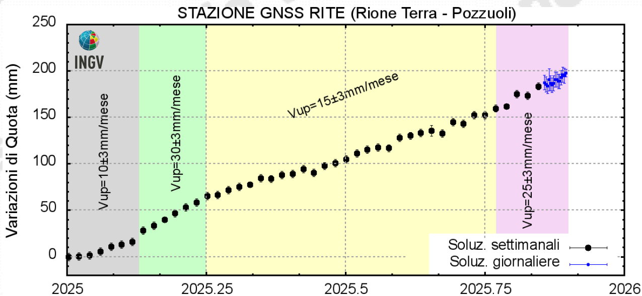
Figura 4.2 – Serie temporale delle variazioni in quota della stazione GNSS di RITE dal 01/01/2025 al 23/11/2025. Elaborazione dati in modalità differenziale singola baseline con software GNSS Spider.
