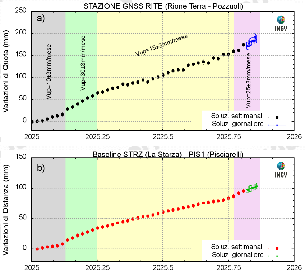
Figura 4.2 – a) Serie temporale delle variazioni in quota della stazione GNSS di RITE dal 01/01/2025 al 09/11/2025; b) Serie temporale delle variazioni di distanza (baseline) tra le stazioni GNSS di STRZ e PIS1 dal 01/01/2025 al 09/11/2025.
