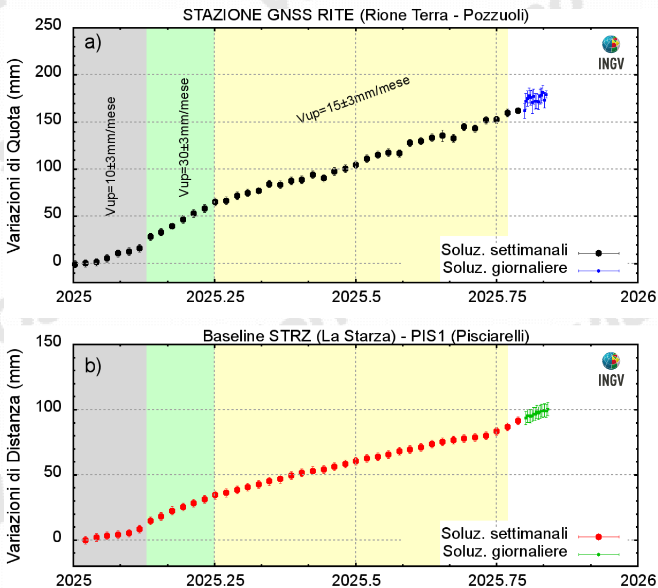
Figura 4.2 – a) Serie temporale delle variazioni in quota della stazione GNSS di RITE dal 01/01/2025 al 02/11/2025; b) Serie temporale delle variazioni di distanza (baseline) tra le stazioni GNSS di STRZ e PIS1 dal 01/01/2025 al 02/11/2025.
