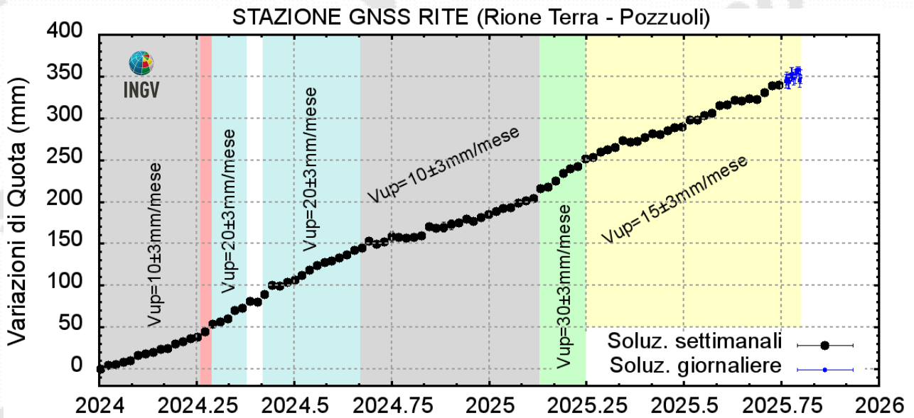
Figura 4.2 – Serie temporale delle variazioni in quota della stazione GNSS di RITE dal 01/01/2024 al 19/10/2025. Elaborazione dati in modalità differenziale singola baseline con software GNSS Spider.
