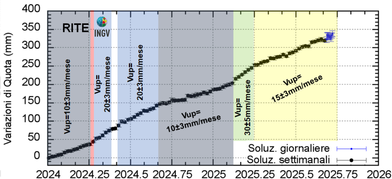
Figura 4.2 – Serie temporale delle variazioni in quota della stazione GNSS di RITE dal 01/01/2024 al 21/09/2025. Elaborazione dati in modalità differenziale singola baseline con software GNSS Spider.
