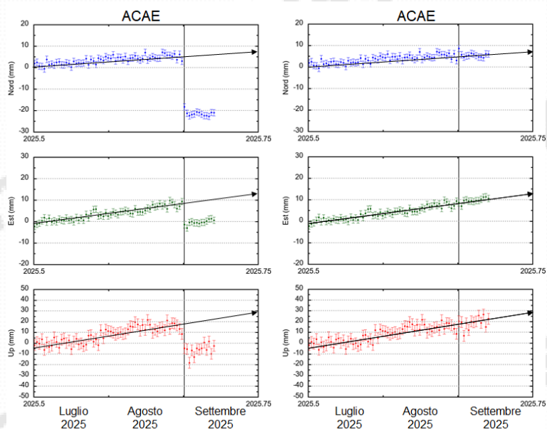
Figura 4.4 - Serie temporali giornaliere della stazione GNSS di ACAE (Accademia Aeronautica) dal 01/01/2024 al 14/09/2025 (Elaborazione dati con software GNSS Bernese). Le linee nere verticali indicano la data del 01/09/2025. Le frecce nere indicano i trend di deformazione calcolati con i dati dei mesi di luglio e agosto 2025.
