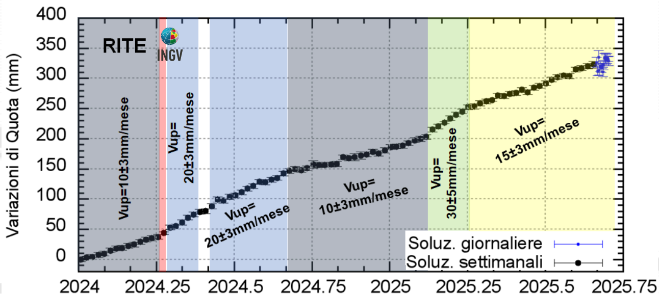
Figura 4.2 – Serie temporale delle variazioni in quota della stazione GNSS di RITE dal 01/01/2024 al 14/09/2025. Elaborazione dati in modalità differenziale singola baseline con software GNSS Spider.
