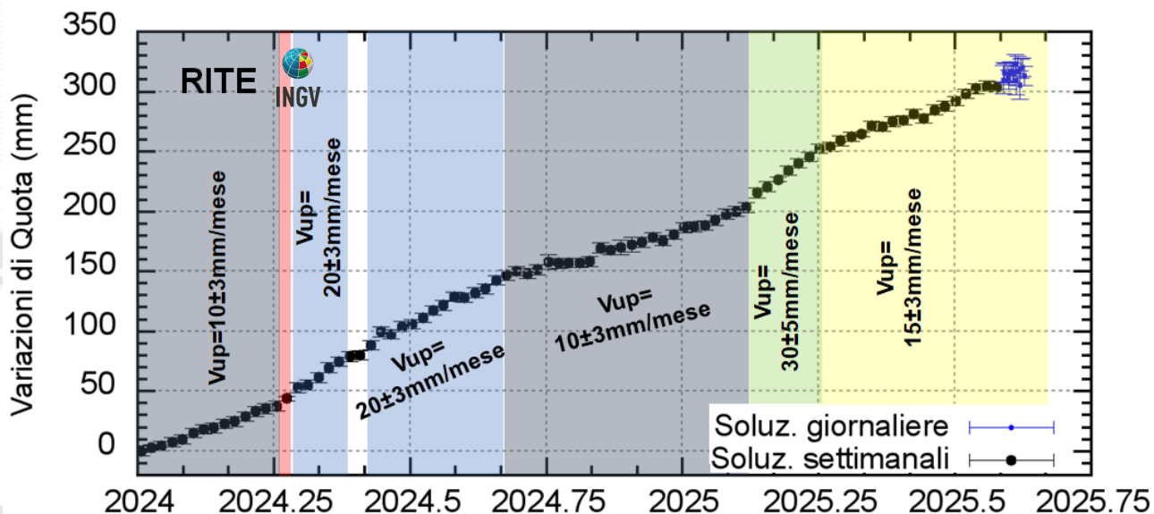
Figura 4.2 – Serie temporale delle variazioni in quota della stazione GNSS di RITE dal 01/01/2024 al 17/08/2025. Elaborazione dati in modalità differenziale singola baseline con software GNSS Spider.
