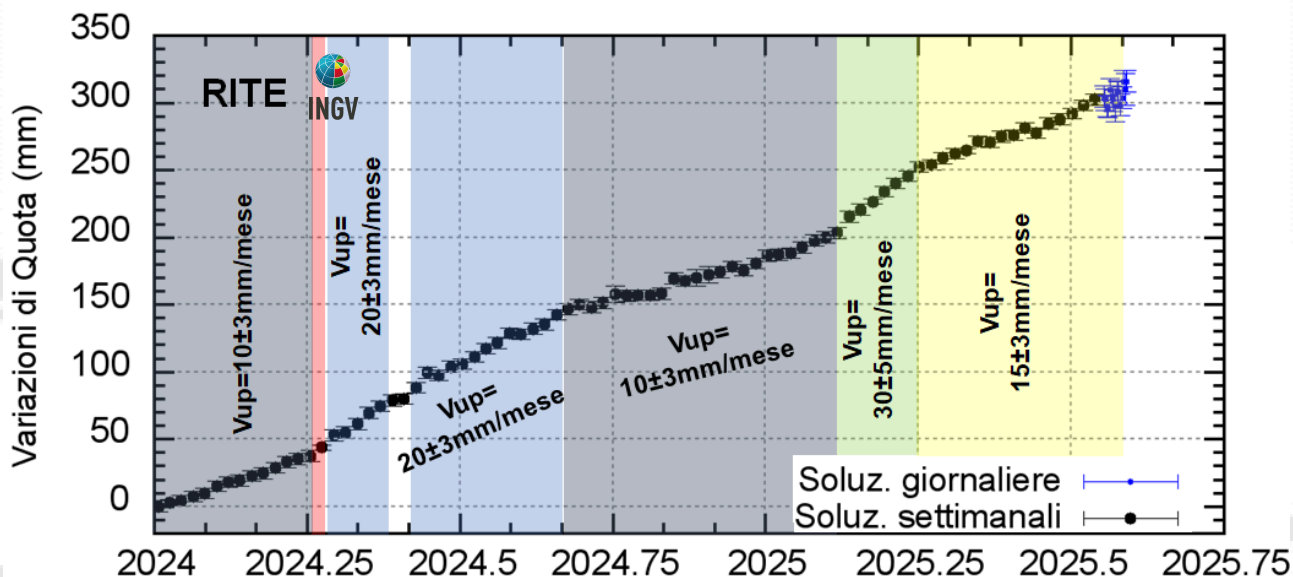
Figura 4.2 – Serie temporale delle variazioni in quota della stazione GNSS di RITE dal 01/01/2024 al 04/08/2025. Elaborazione dati in modalità differenziale singola baseline con software GNSS Spider.
