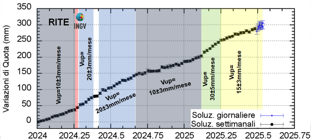
Figura 4.2 – Serie temporale delle variazioni in quota della stazione GNSS di RITE dal 01/01/2024 al 14/07/2025. Elaborazione dati in modalità differenziale singola baseline con software GNSS Spider.
