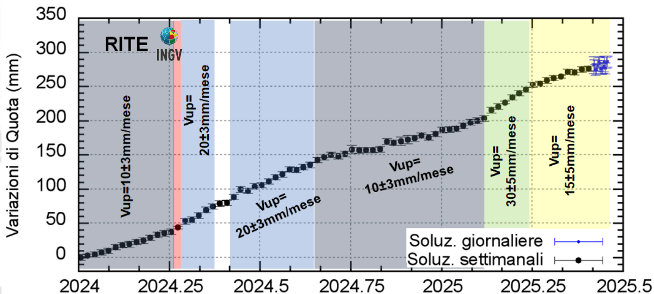
Figura 4.2 – Serie temporale delle variazioni in quota della stazione GNSS di RITE dal 01/01/2024 al 16/06/2025. Elaborazione dati in modalità differenziale singola baseline con software GNSS Spider.
