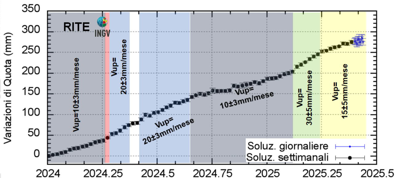
Figura 4.2 – Serie temporale delle variazioni in quota della stazione GNSS di RITE dal 01/01/2024 al 09/06/2025. Elaborazione dati in modalità differenziale singola baseline con software GNSS Spider.
