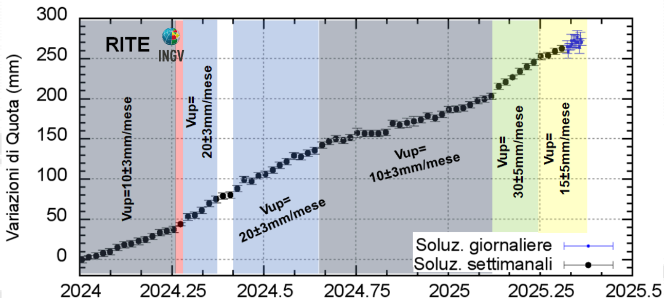
Figura 4.2 – Serie temporale delle variazioni in quota della stazione GNSS di RITE dal 01/01/2024 al 12/05/2025. Elaborazione dati in modalità differenziale singola baseline con software GNSS Spider.
