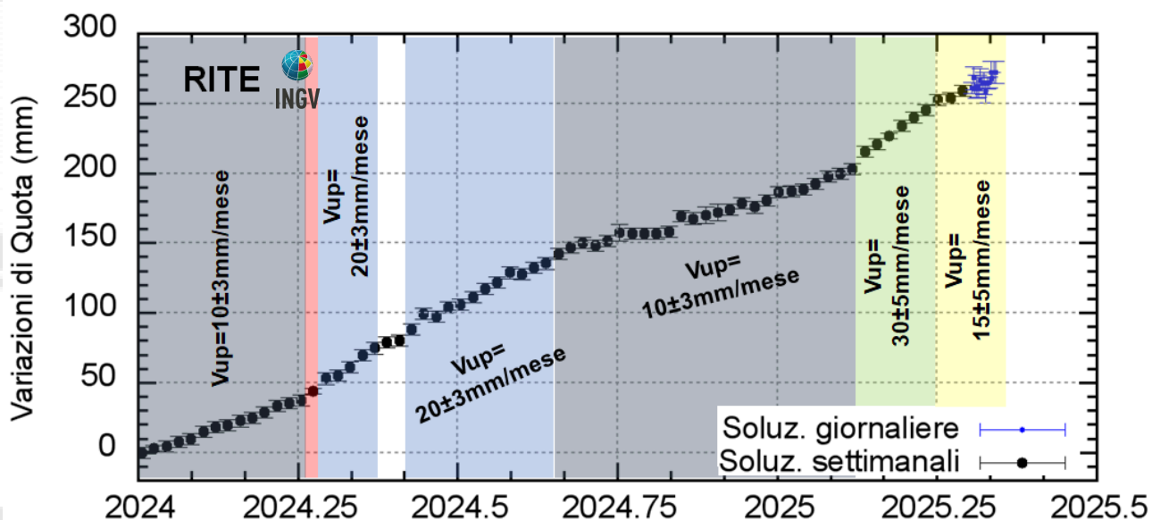
Figura 4.2 – Serie temporale delle variazioni in quota della stazione GNSS di RITE dal 01/01/2024 al 05/05/2025. Elaborazione dati in modalità differenziale singola baseline con software GNSS Spider.
