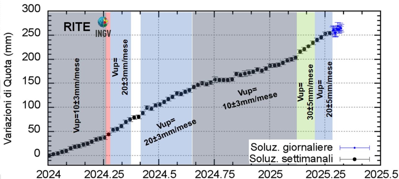
Figura 4.2 – Serie temporale delle variazioni in quota della stazione GNSS di RITE dal 01/01/2024 al 28/04/2025. Elaborazione dati in modalità differenziale singola baseline con software GNSS Spider.
