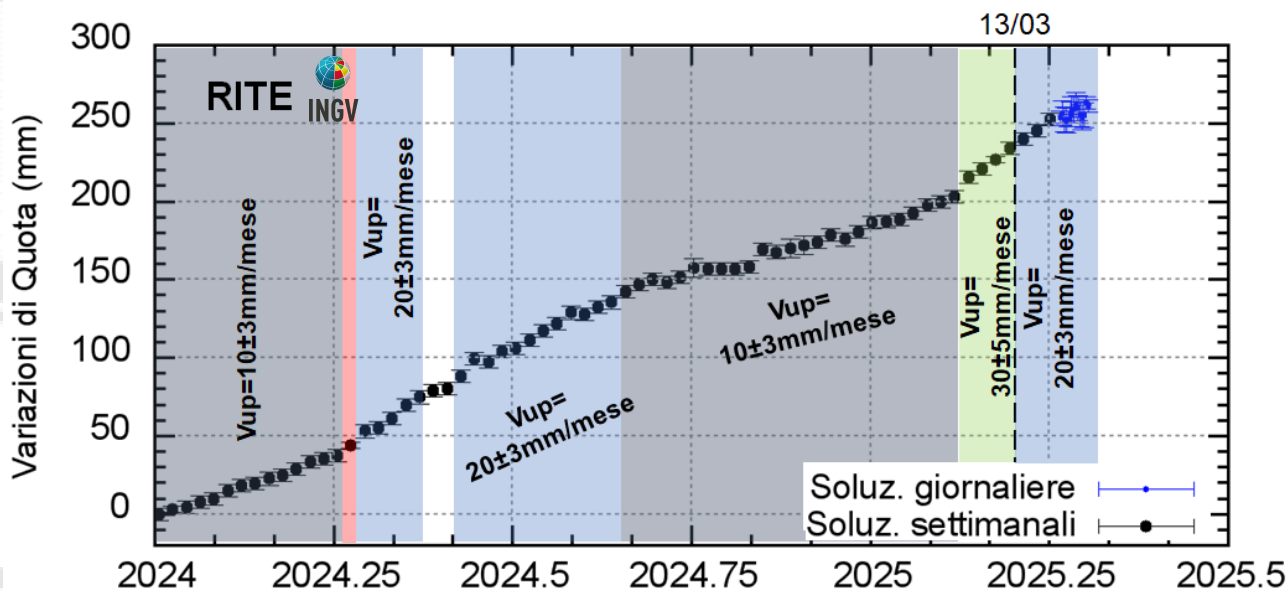
Figura 4.2 – Serie temporale delle variazioni in quota della stazione GNSS di RITE dal 01/01/2024 al 21/04/2025. Elaborazione dati in modalità differenziale singola baseline con software GNSS Spider.
