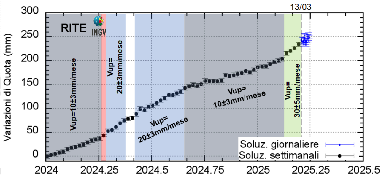
Figura 4.2 – Serie temporale delle variazioni in quota della stazione GNSS di RITE dal 01/01/2024 al 31/03/2025. Elaborazione dati in modalità differenziale singola baseline con software GNSS Spider.
