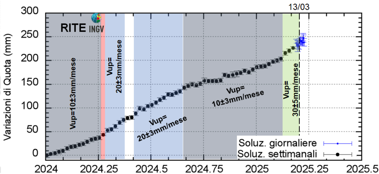
Figura 4.2 – Serie temporale delle variazioni in quota della stazione GNSS di RITE dal 01/01/2024 al 24/03/2025. Elaborazione dati in modalità differenziale singola baseline con software GNSS Spider.
