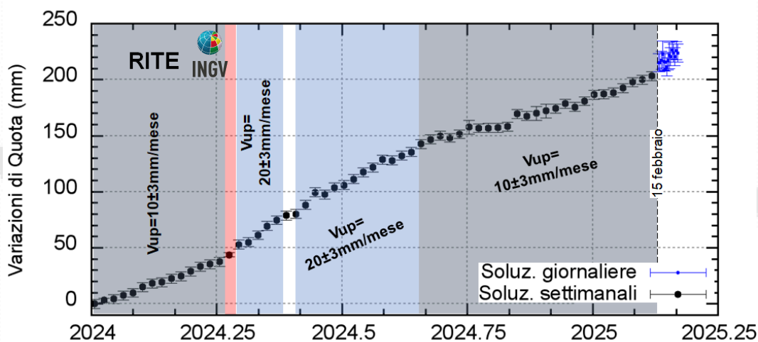
Figura 4.2 - Serie temporale delle variazioni in quota della stazione GNSS di RITE dal 01/01/2024 al 03/03/2025. Elaborazione dati in modalità differenziale singola baseline con software GNSS Spider.
