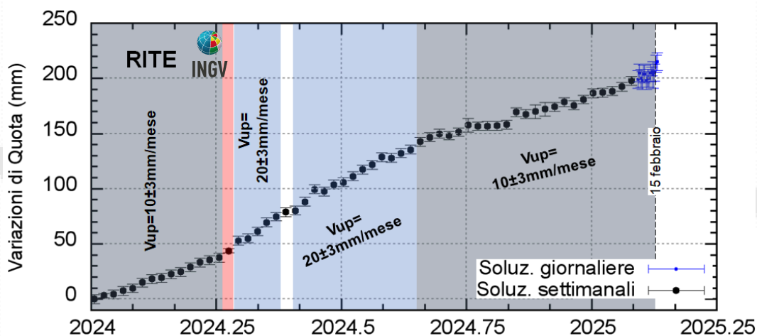
Figura 4.2 - Serie temporale delle variazioni in quota della stazione GNSS di RITE dal 01/01/2024 al 17/02/2025. Elaborazione dati in modalità differenziale singola baseline con software GNSS Spider.
