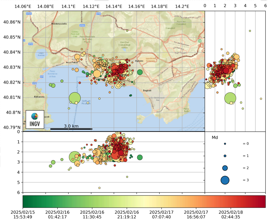
Figura 3.2 - Ipocentri dei terremoti con magnitudo M_d \geq 0.0 localizzati durante lo sciame iniziato alle 15:53 UTC del 15 febbraio 2025 e tuttora in corso.
