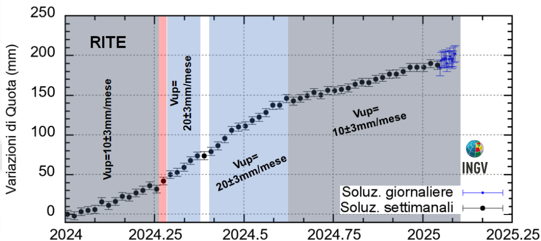
Figura 4.2 - Serie temporale delle variazioni in quota della stazione GNSS di RITE dal 01/01/2024 al 02/02/2025. Elaborazione dati in modalità Precise Point Positioning con software PRIDE PPP-AR.
