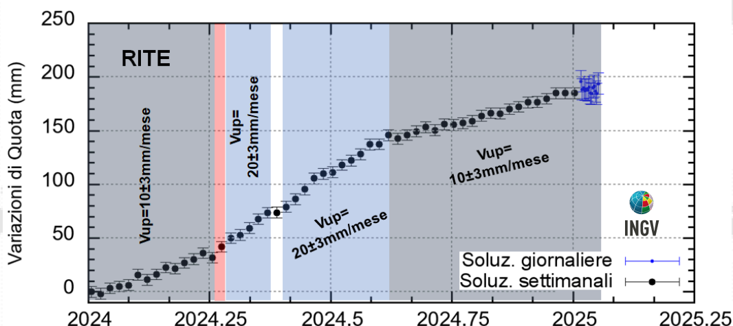
Figura 4.2 - Serie temporale delle variazioni in quota della stazione GNSS di RITE dal 01/01/2024 al 19/01/2025. Elaborazione dati in modalità Precise Point Positioning con software PRIDE PPP-AR.
