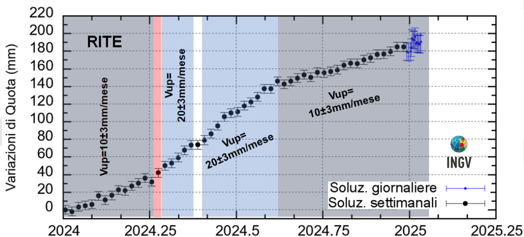
Figura 4.2 - Serie temporale delle variazioni in quota della stazione GNSS di RITE dal 01/01/2024 al 12/01/2025. Elaborazione dati in modalità Precise Point Positioning con software PRIDE PPP-AR.
