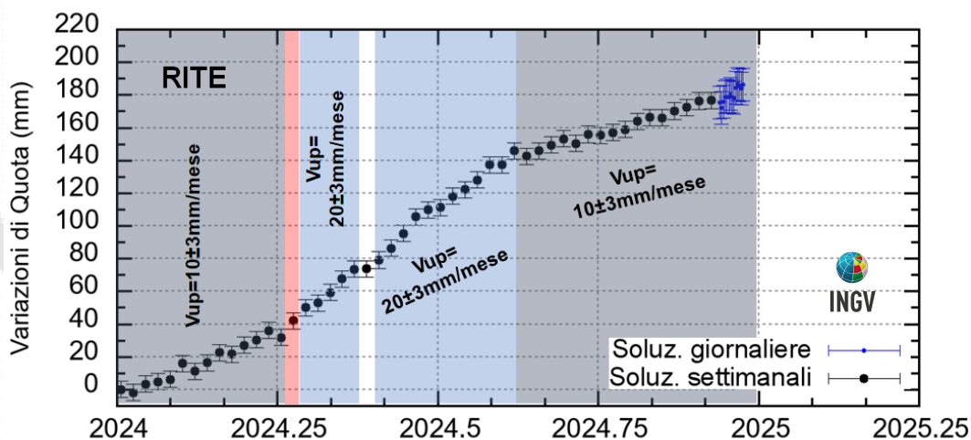
Figura 4.2 - Serie temporale delle variazioni in quota della stazione GNSS di RITE dal 01/01/2024 al 22/12/2024. Elaborazione dati in modalità Precise Point Positioning con software PRIDE PPP-AR.
