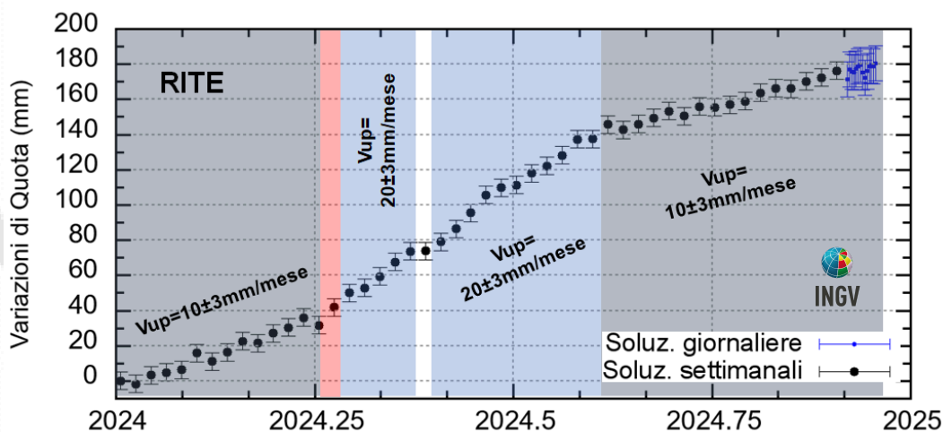
Figura 4.2 - Serie temporale delle variazioni in quota della stazione GNSS di RITE dal 01/01/2024 al 15/12/2024. Elaborazione dati in modalità Precise Point Positioning con software PRIDE PPP-AR.
