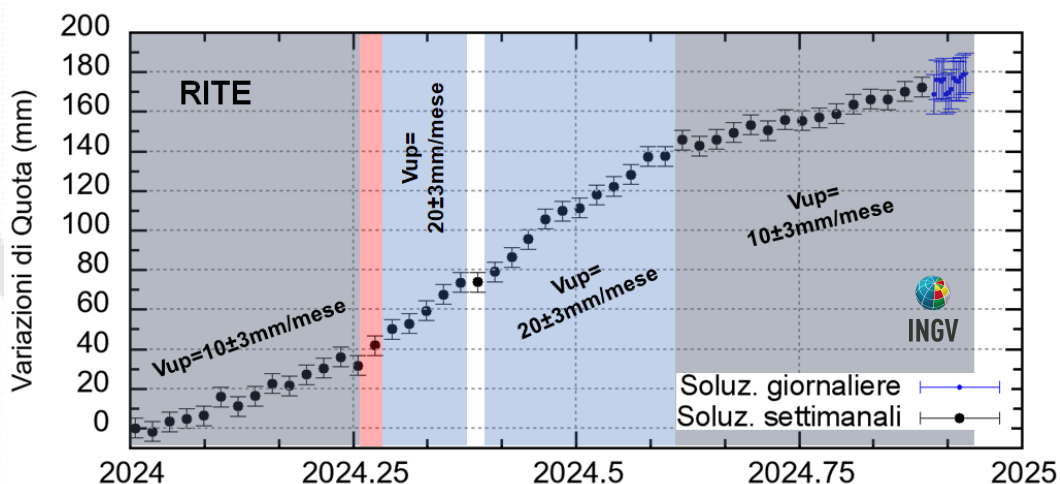
Figura 4.2 - Serie temporale delle variazioni in quota della stazione GNSS di RITE dal 01/01/2024 al 08/12/2024. Elaborazione dati in modalità Precise Point Positioning con software PRIDE PPP-AR.
