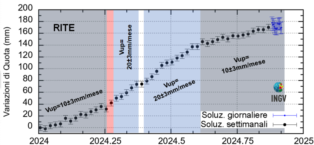
Figura 4.2 - Serie temporale delle variazioni in quota della stazione GNSS di RITE dal 01/01/2024 al 01/12/2024. Elaborazione dati in modalità Precise Point Positioning con software PRIDE PPP-AR.
