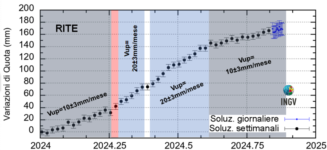
Figura 4.2 - Serie temporale delle variazioni in quota della stazione GNSS di RITE dal 01/01/2024 al 17/11/2024. Elaborazione dati in modalità Precise Point Positioning con software PRIDE PPP-AR.
