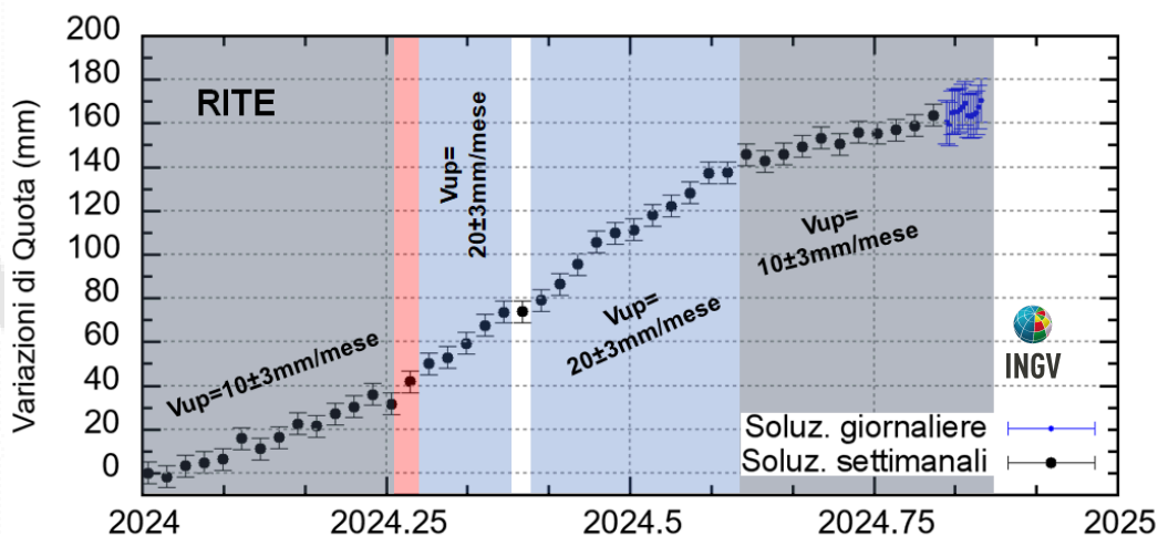
Figura 4.2 - Serie temporale delle variazioni in quota della stazione GNSS di RITE dal 01/01/2024 al 10/11/2024. Elaborazione dati in modalità Precise Point Positioning con software PRIDE PPP-AR.
