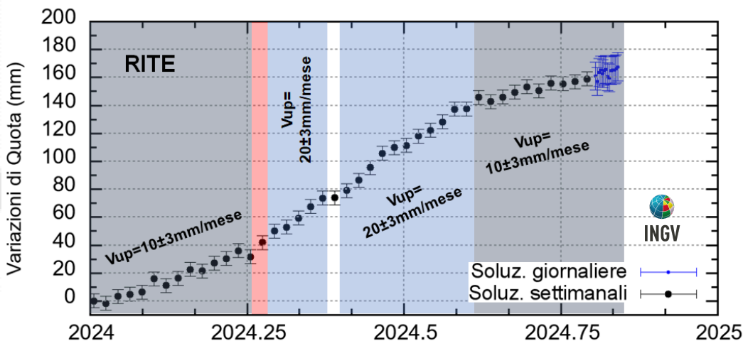
Figura 4.2 - Serie temporale delle variazioni in quota della stazione GNSS di RITE dal 01/01/2024 al 03/11/2024. Elaborazione dati in modalità Precise Point Positioning con software PRIDE PPP-AR.
