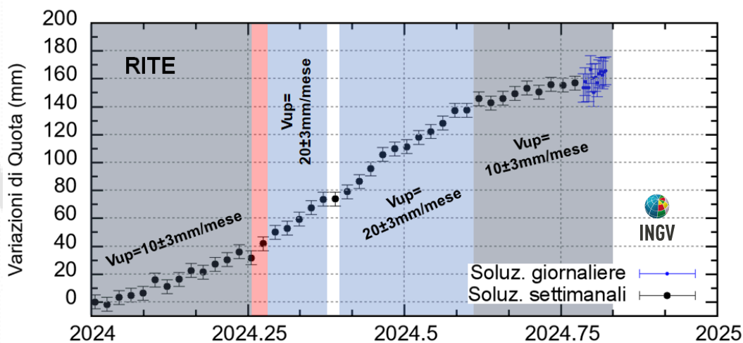
Figura 4.2 - Serie temporale delle variazioni in quota della stazione GNSS di RITE dal 01/01/2024 al 27/10/2024. Elaborazione dati in modalità Precise Point Positioning con software PRIDE PPP-AR.
