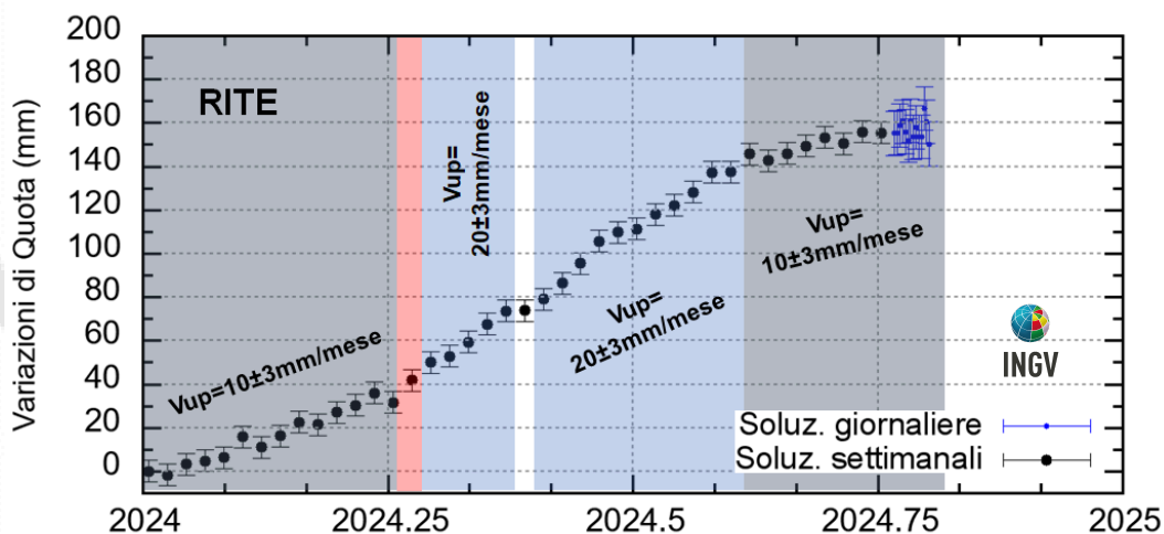
Figura 4.2 - Serie temporale delle variazioni in quota della stazione GNSS di RITE dal 01/01/2024 al 20/10/2024. Elaborazione dati in modalità Precise Point Positioning con software PRIDE PPP-AR.
