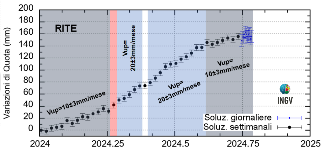
Figura 4.2 - Serie temporale delle variazioni in quota della stazione GNSS di RITE dal 01/01/2024 al 13/10/2024. Elaborazione dati in modalità Precise Point Positioning con software PRIDE PPP-AR.
