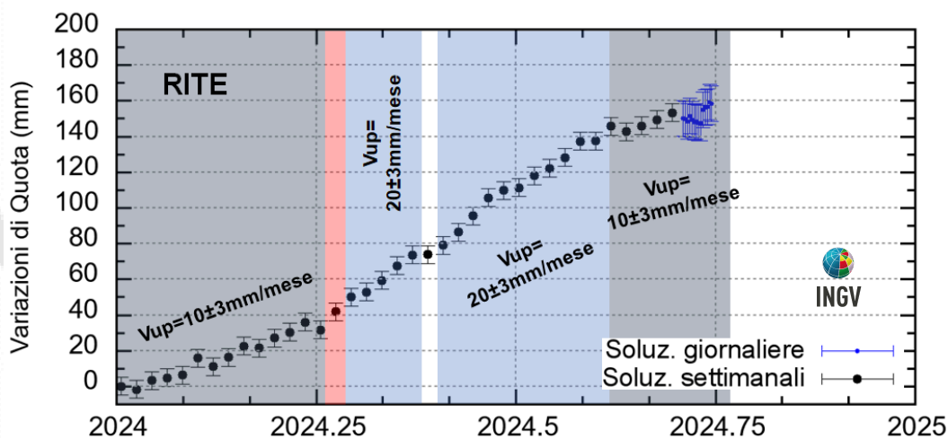
Figura 4.2 - Serie temporale delle variazioni in quota della stazione GNSS di RITE dal 01/01/2024 al 29/09/2024. Elaborazione dati in modalità Precise Point Positioning con software PRIDE PPP-AR.
