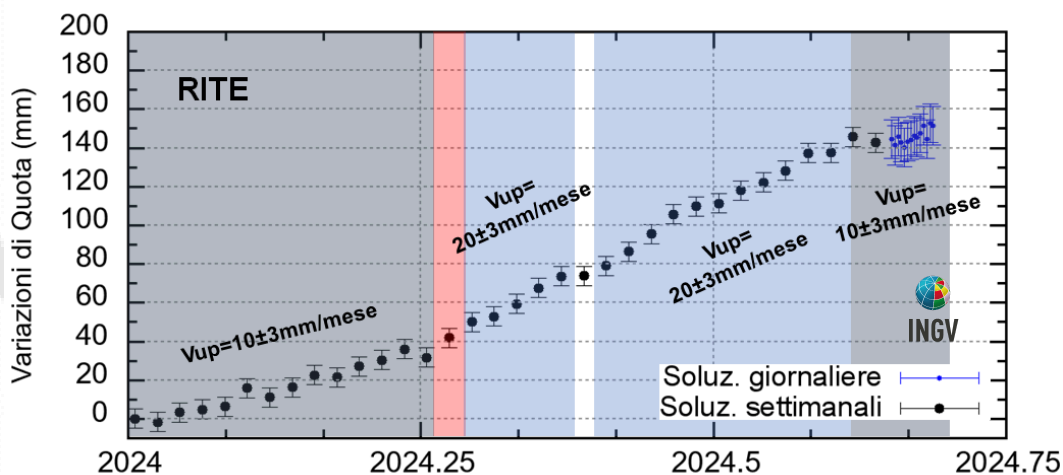
Figura 4.2 - Serie temporale delle variazioni in quota della stazione GNSS di RITE dal 01/01/2024 al 08/09/2024. Elaborazione dati in modalità Precise Point Positioning con software PRIDE PPP-AR.
