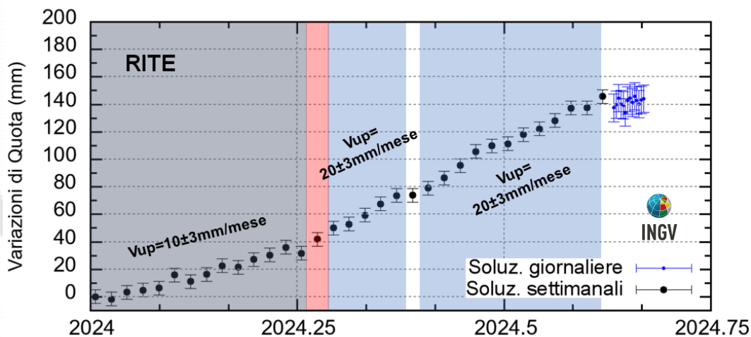
Figura 4.2 - Serie temporale delle variazioni in quota della stazione GNSS di RITE dal 01/01/2024 al 01/09/2024. Elaborazione dati in modalità Precise Point Positioning con software PRIDE PPP-AR.
