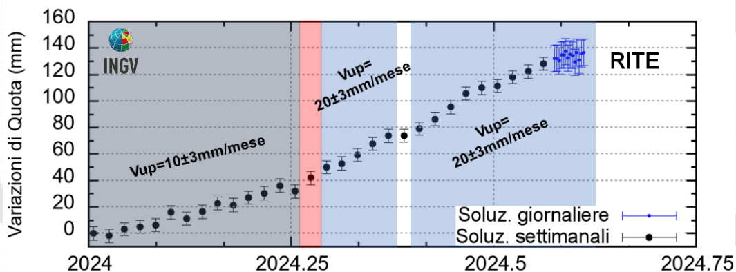
Figura 4.2 - Serie temporale delle variazioni in quota della stazione GNSS di RITE dal 01/01/2024 al 11/08/2024. Elaborazione dati in modalità Precise Point Positioning con software PRIDE PPP-AR.
