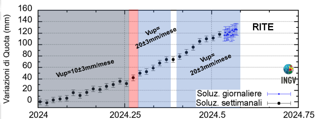
Figura 4.2 - Serie temporale delle variazioni in quota della stazione GNSS di RITE dal 01/01/2024 al 28/07/2024. Elaborazione dati in modalità Precise Point Positioning con software PRIDE PPP-AR.
