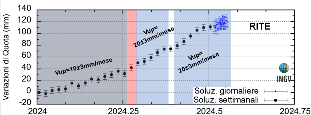
Figura 4.2 - Serie temporale delle variazioni in quota della stazione GNSS di RITE dal 01/01/2024 al 21/07/2024. Elaborazione dati in modalità Precise Point Positioning con software PRIDE PPP-AR.
