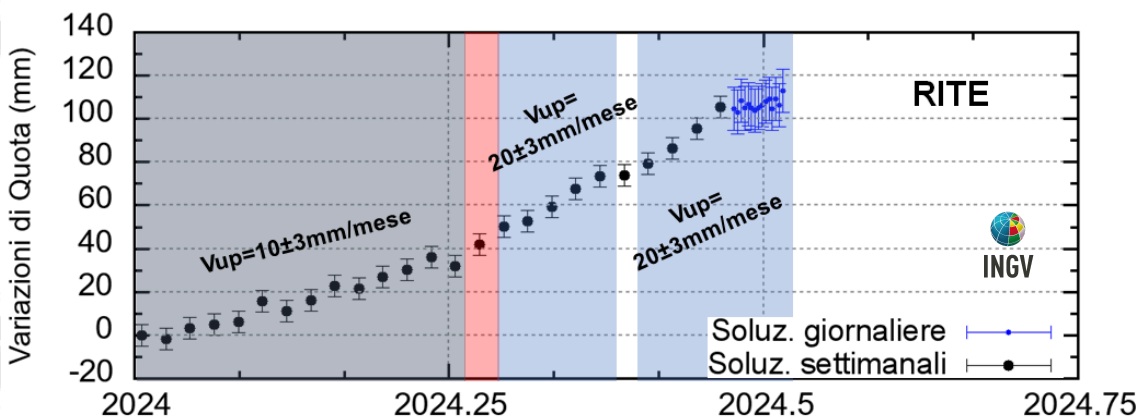
Figura 4.2 - Serie temporale delle variazioni in quota della stazione GNSS di RITE dal 01/01/2024 al 07/07/2024. Elaborazione dati in modalità Precise Point Positioning con software PRIDE PPP-AR.
