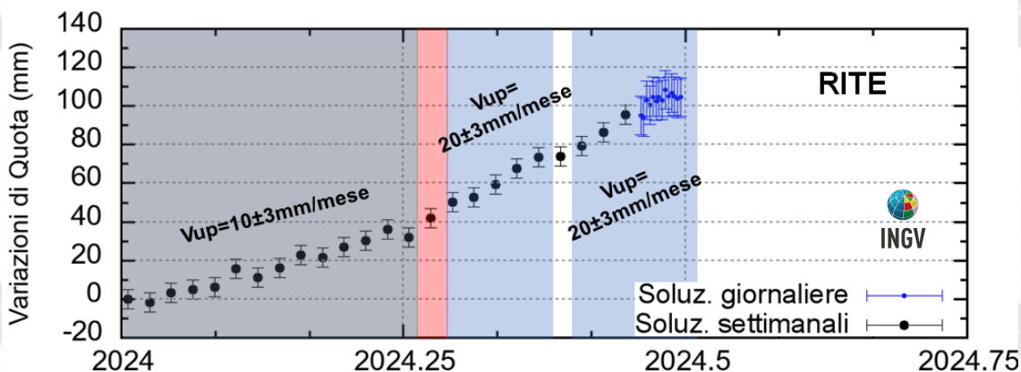
Figura 4.2 - Serie temporale delle variazioni in quota della stazione GNSS di RITE dal 01/01/2024 al 30/06/2024. Elaborazione dati in modalità Precise Point Positioning con software PRIDE PPP-AR.
