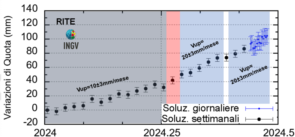
Figura 4.2 - Serie temporale delle variazioni in quota della stazione GNSS di RITE dal 01/01/2024 al 23/06/2024. Elaborazione dati in modalità Precise Point Positioning con software PRIDE PPP-AR.
