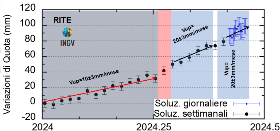
Figura 4.2 - Serie temporale delle variazioni in quota della stazione GNSS di RITE dal 01/01/2024 al 16/06/2024. Elaborazione dati in modalità Precise Point Positioning con software PRIDE PPP-AR.
