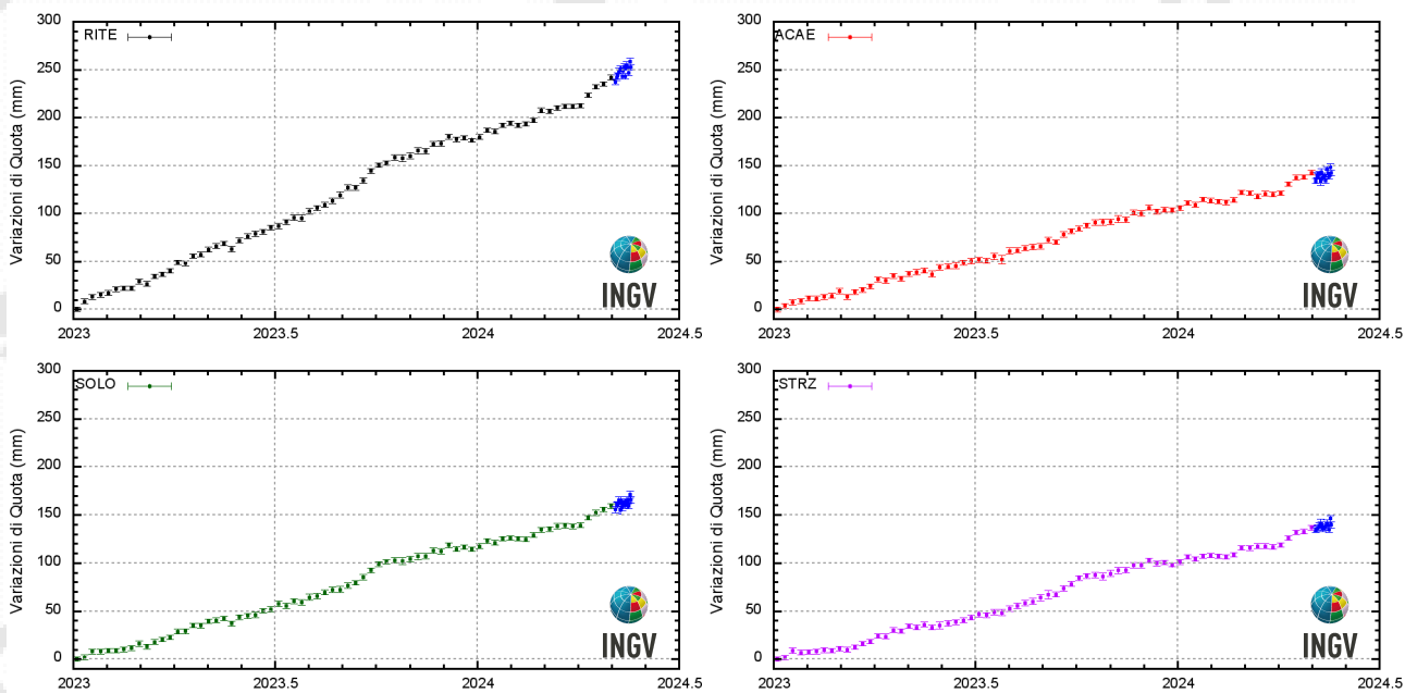
Figura 4.4 - Serie temporali delle variazioni in quota delle stazioni di RITE (Pozzuoli – Rione Terra), ACAE (Accademia Aeronautica), SOLO (Solfatara) e STRZ (Pozzuoli - Cimitero) dal 01/01/2023 al 19/05/2024.
