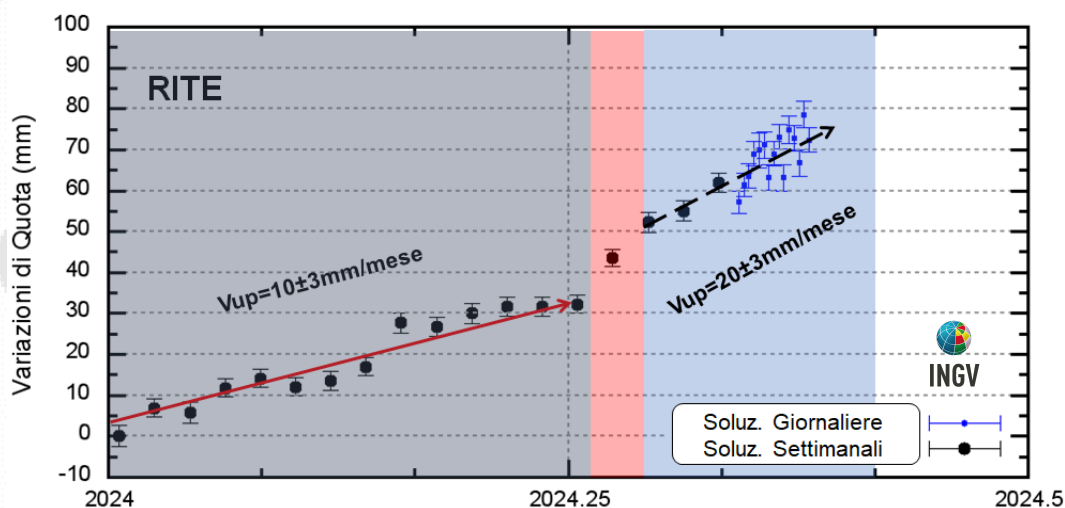
Figura 4.3 - Serie temporale delle variazioni in quota della stazione GNSS di RITE dal 01/01/2024 al 19/05/2024.
