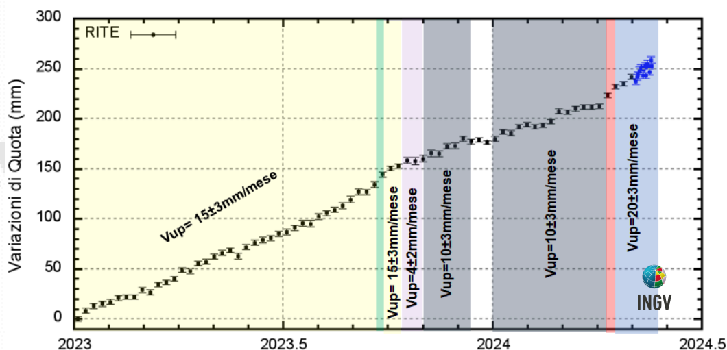
Figura 4.2 - Serie temporale delle variazioni in quota della stazione GNSS di RITE dal 01/01/2023 al 19/05/2024.
