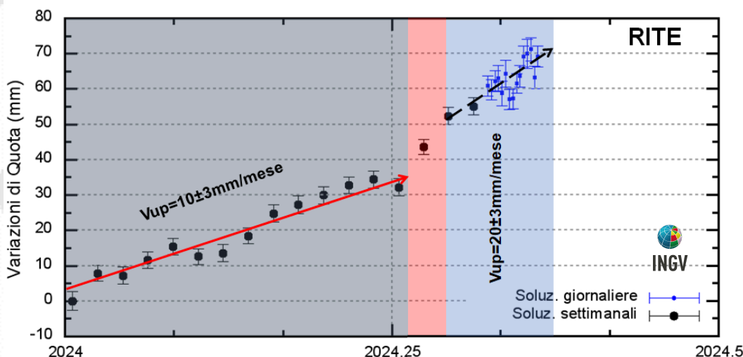
Figura 4.3 - Serie temporale delle variazioni in quota della stazione GNSS di RITE dal 01/01/2024 al 12/05/2024.
