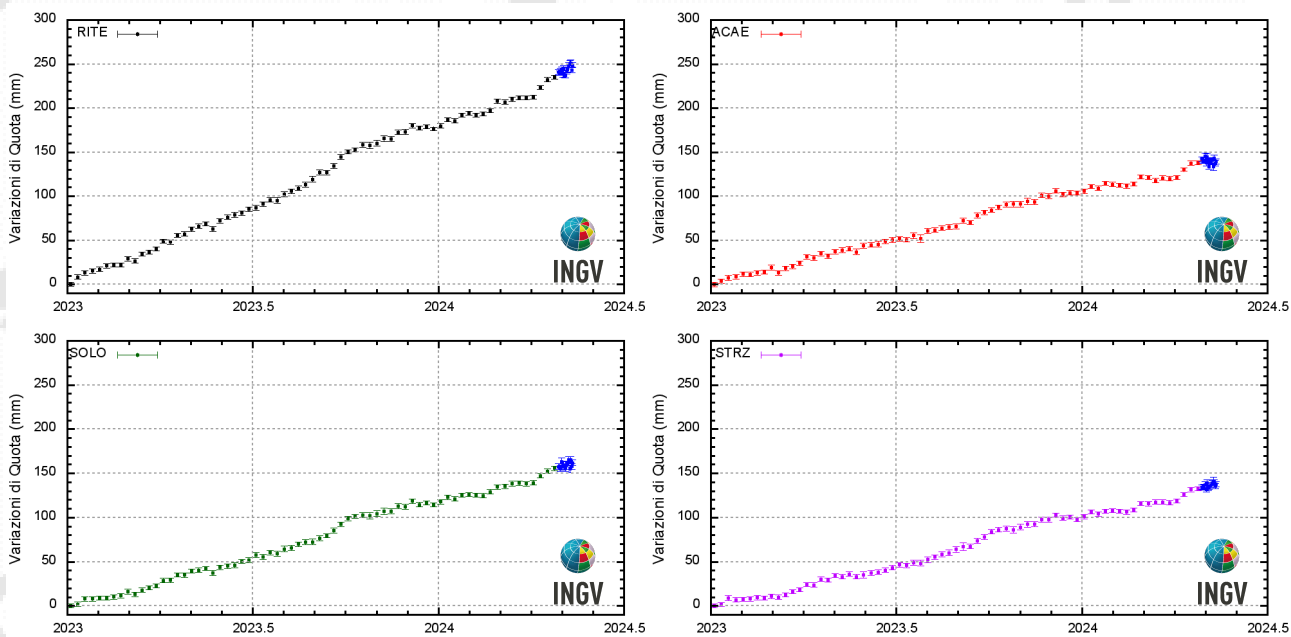
Figura 4.4 - Serie temporali delle variazioni in quota delle stazioni di RITE (Pozzuoli – Rione Terra), ACAE (Accademia Aeronautica), SOLO (Solfatara) e STRZ (Pozzuoli - Cimitero) dal 01/01/2023 al 12/05/2024.
