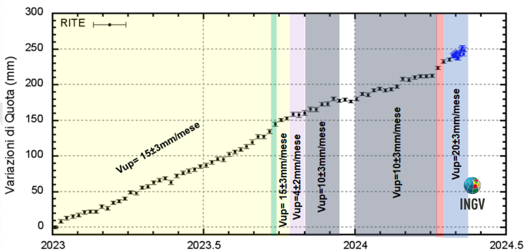
Figura 4.2 - Serie temporale delle variazioni in quota della stazione GNSS di RITE dal 01/01/2023 al 12/05/2024.
