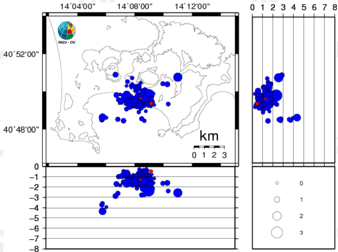
Figura 3.1 - Ipocentri dei terremoti localizzati ai Campi Flegrei negli ultimi 12 mesi (in totale 547). In rosso gli eventi localizzati nell'ultima settimana (in totale 2).
